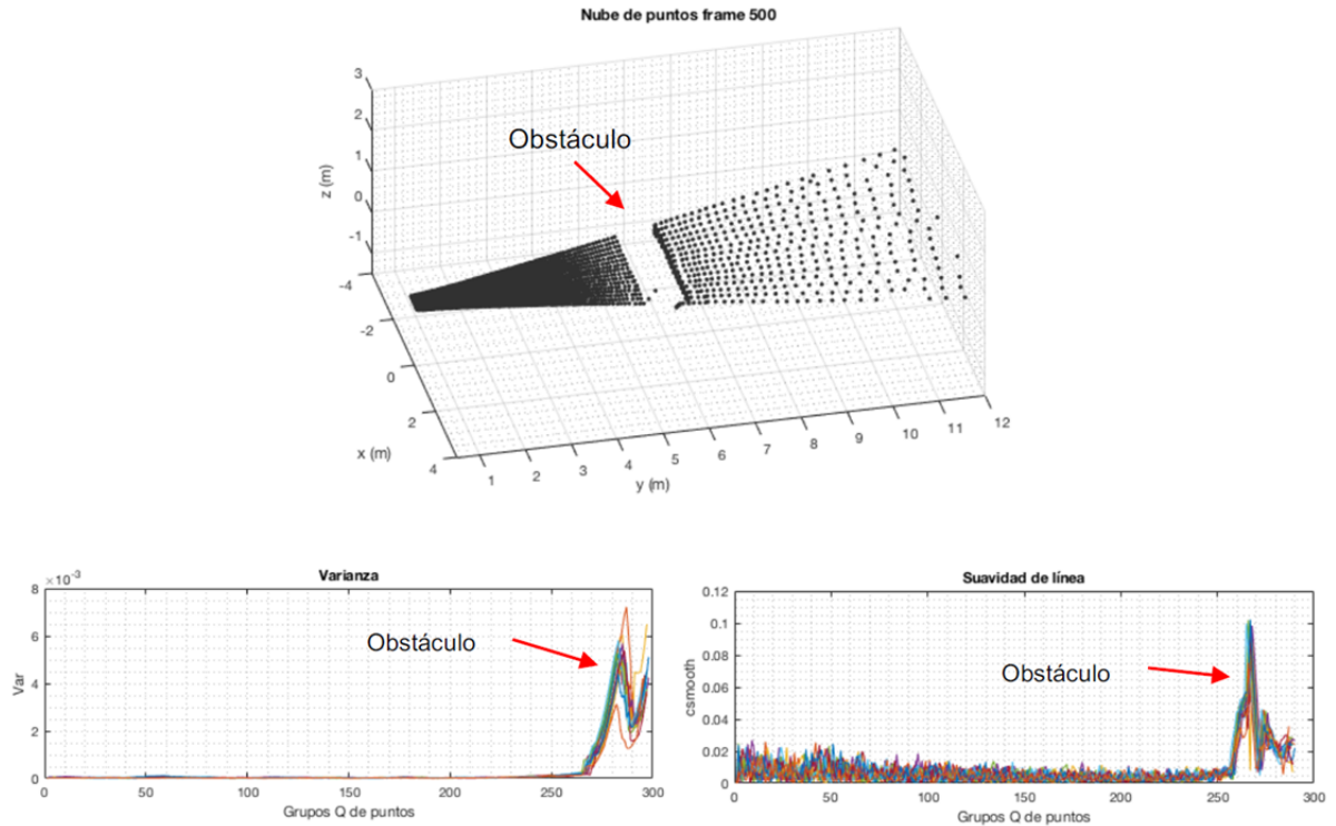
Fig. 4. Comportamiento filtros de identificación ante un obstáculo (representación de las variables en cada capa del LiDAR).
