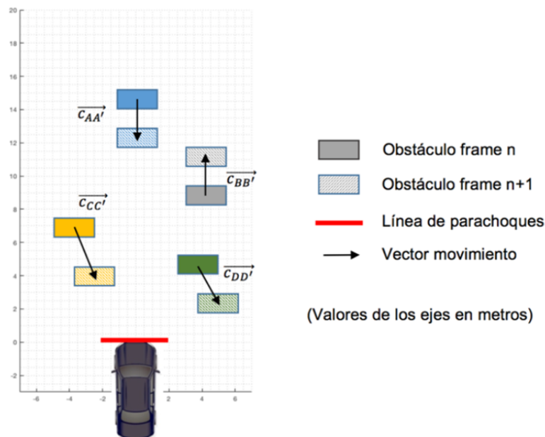
Fig. 6. Tracking de obstáculos.
