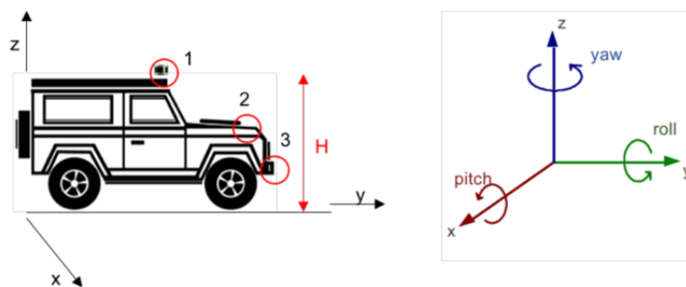
Fig. 1. Posibles instalaciones del LiDAR y los ángulos de orientación.
