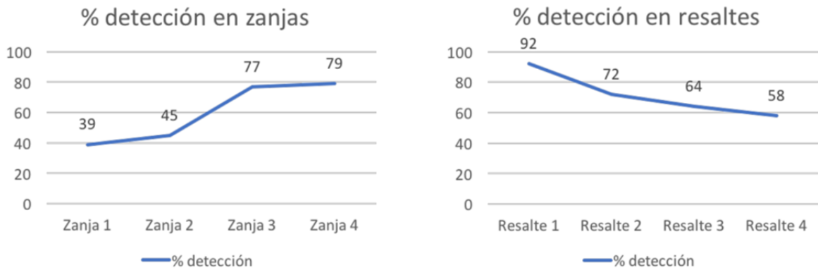
Fig. 10. Precisión detección obstáculos zanjas y resaltes.
